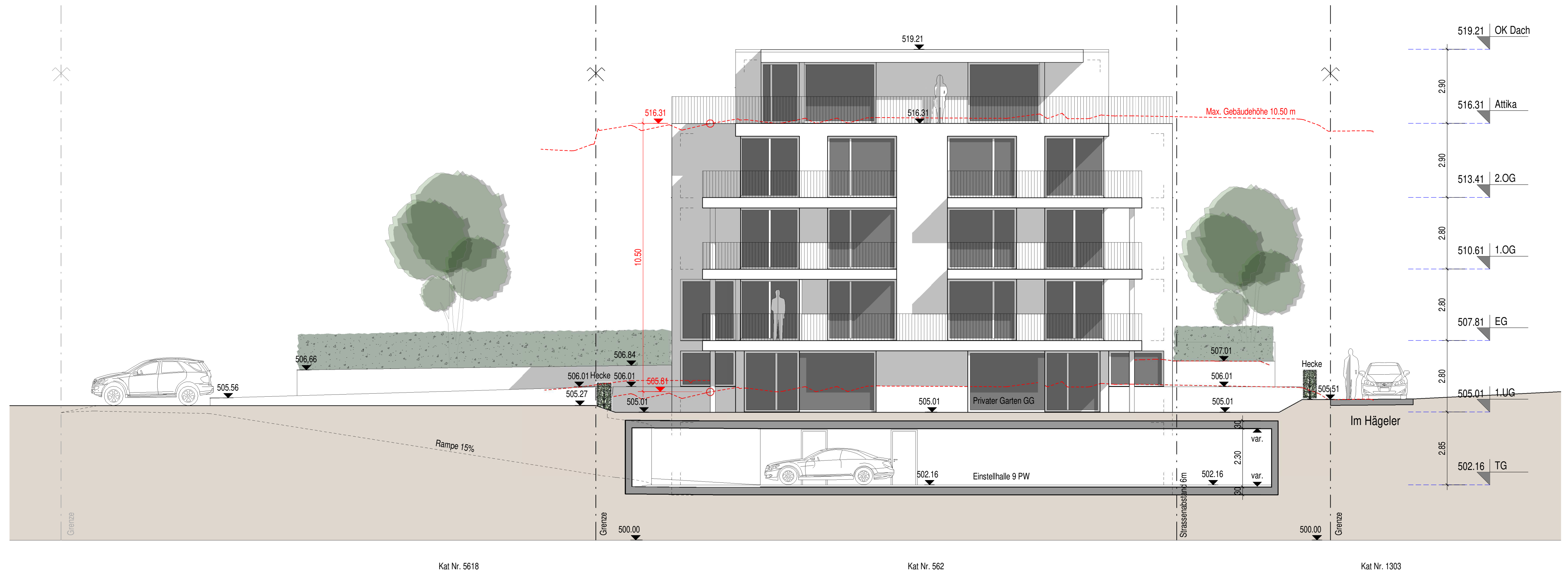
Südwestfassade
