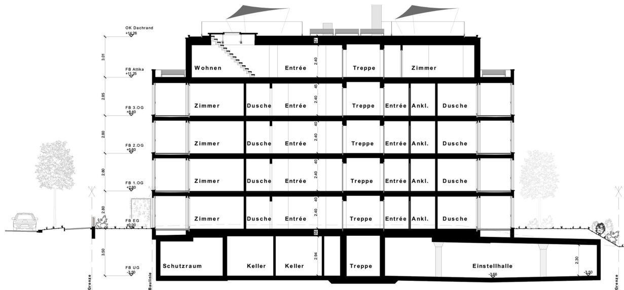
Längsschnitt B
