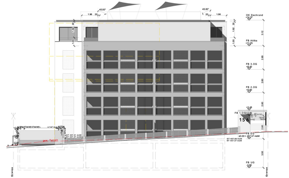
Ansicht Süd
