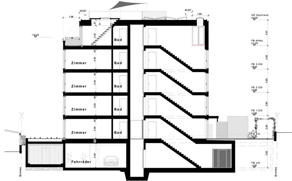
Querschnitt A
