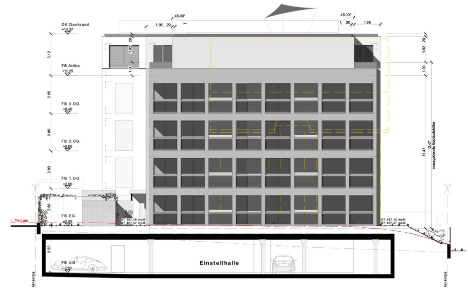
Ansicht Nord
